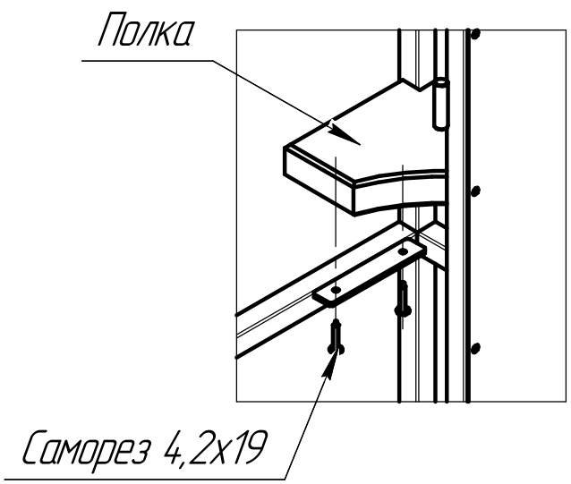
Крепление полки к раме
