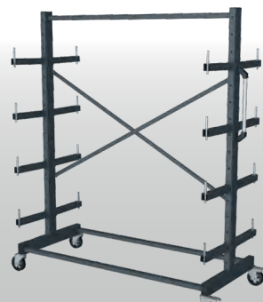
Стеллаж на колесах, двухсторонний ШхГхВ: 1500х650х1835 мм Нагрузка общая: 400 кг Нагрузка на пару консолей: до 100 кг Рабочая глубина консоли: 300 мм Артикул: 1620.504
