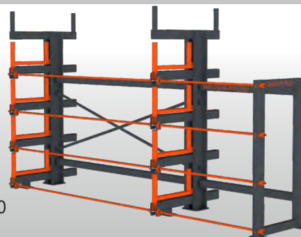
Артикул: 16104.300 для грузов до 6 м 5 полок г/п 3 тн общая г/п 15 тн
